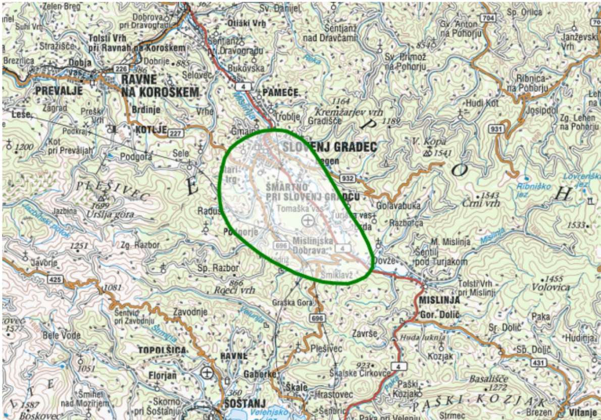
Slika 2: Območje pokrivanja radijske frekvence Slovenj Gradec 105,4 MHz (sklop Slovenj Gradec)
