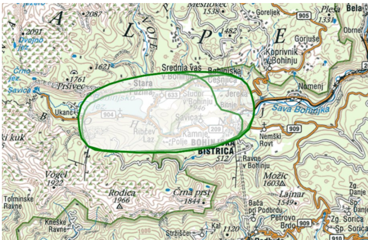
Slika 7: Unija območij pokrivanja radijskih frekvenc na sklopu Bohinj
