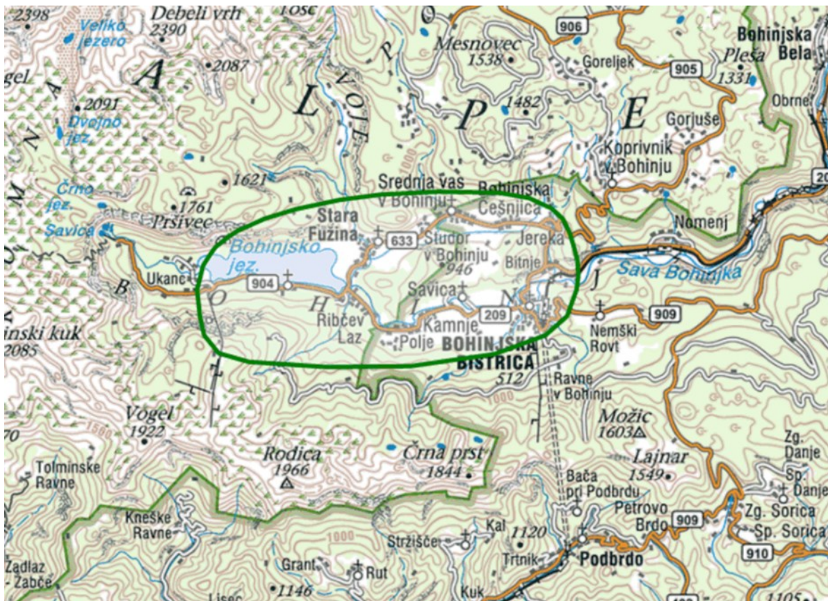
Slika 3: Območje pokrivanja radijske frekvence Vogel 92,6 MHz (sklop Bohinj)
