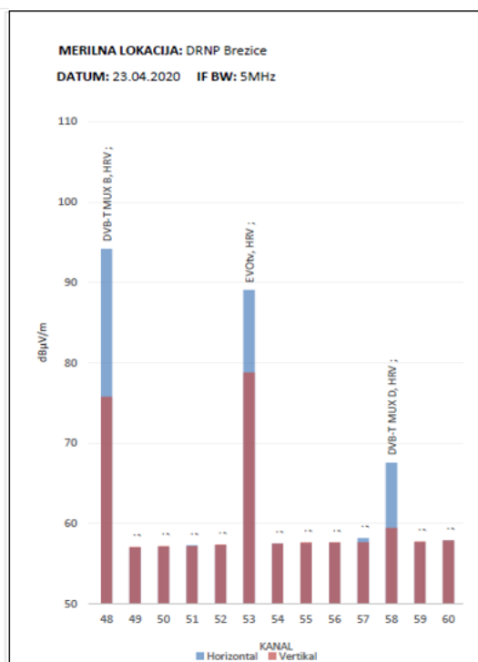
Slika A-8: Meritve zasedenosti spektra z digitalno televizijo DTT v Brežicah – april 2020
