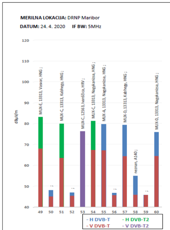
Slika A-9: Meritve zasedenosti spektra z digitalno televizijo DTT v Mariboru – april 2020
