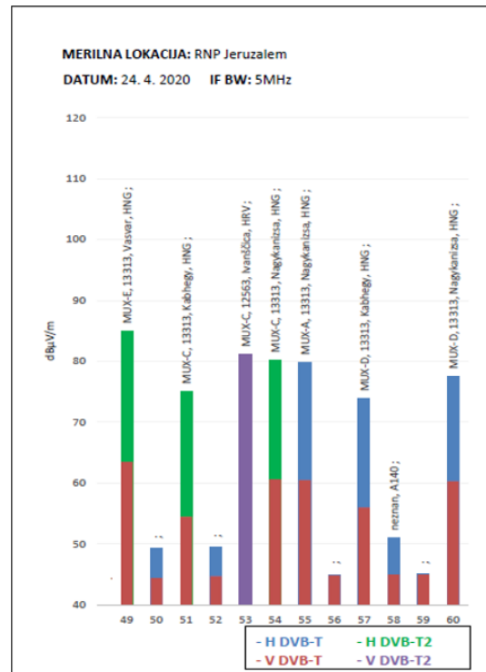
Slika A-10: Meritve zasedenosti spektra z digitalno televizijo DTT in v Jeruzalemu – april 2020
