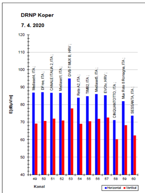
Slika A-11: Meritve zasedenosti spektra z digitalno televizijo DTT in v Kopru – april 2020
