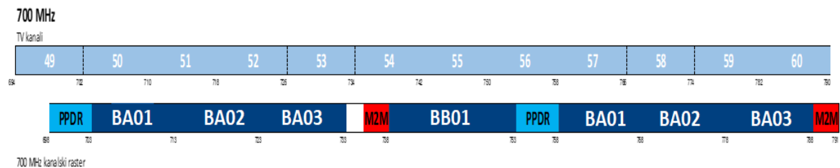
Slika A-3: Primerjava kanalskih rastrov za mobilne in radiodifuzne storitve
