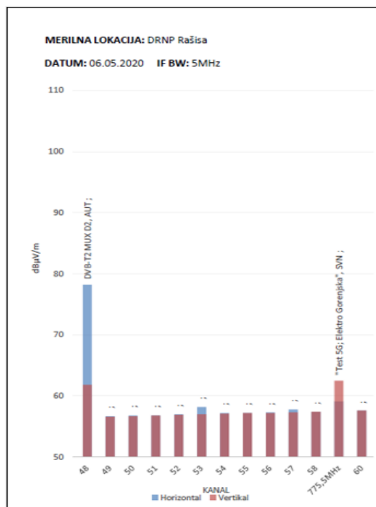
Slika A-7: Meritve zasedenosti spektra z digitalno televizijo DTT v Ljubljani (Rašica) – maj 2020
